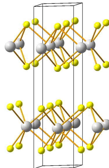
\text{MoS}_2
