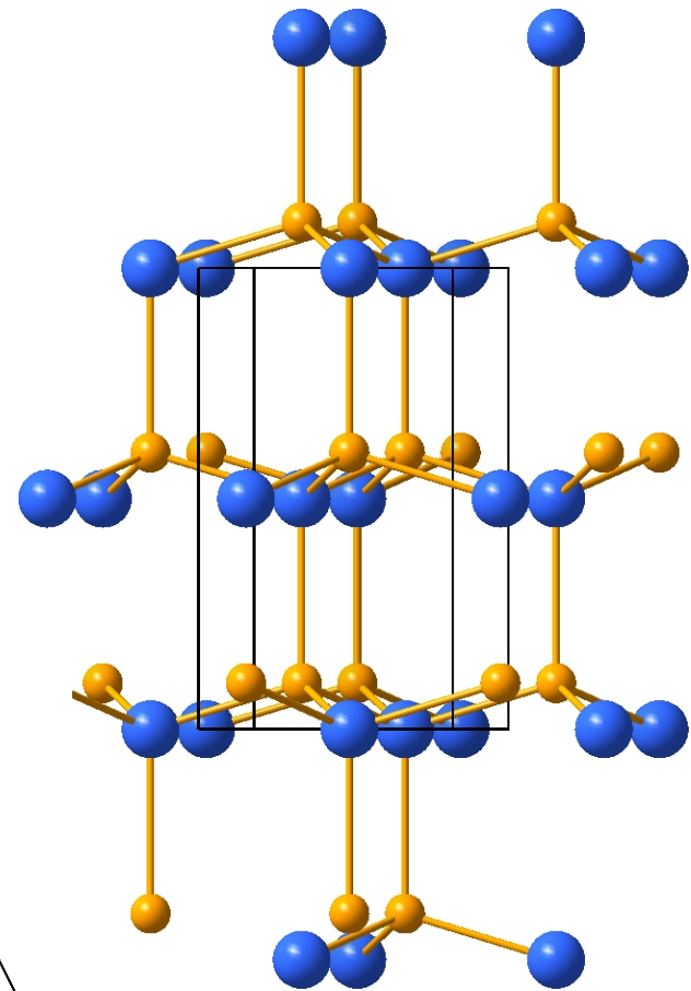
ZnS Wurtzite
