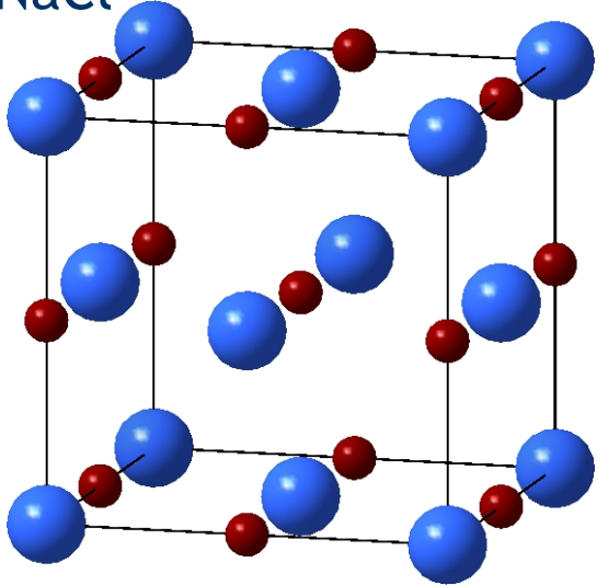
NiAs
