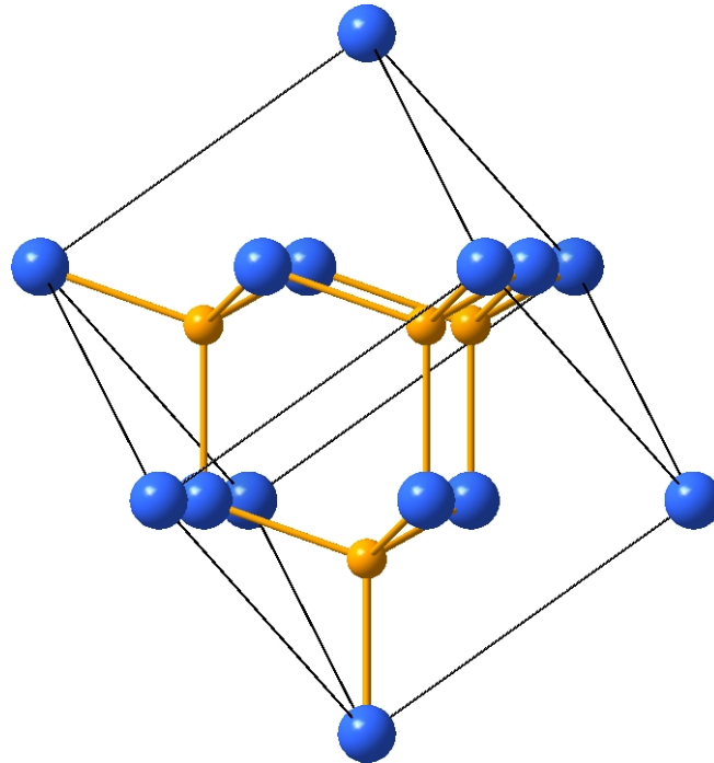
ZnS Blende
