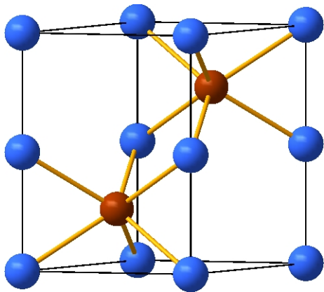
NiAs
